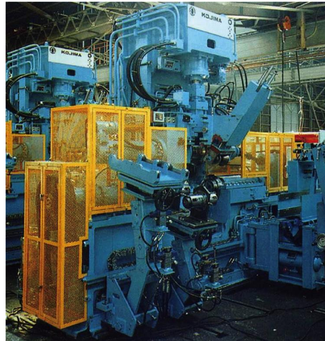
ダブルエンドタイプロールフォーマー Double End Rotary Roll Former
