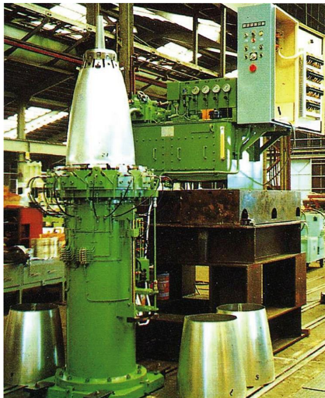
油圧式エキスパンダー Hydraulic Expander
