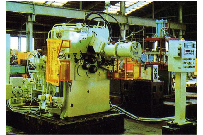
3RCコイラー(リングギヤ素材1本巻用) 3RC Coiler for Ring Gear Blank with Cutter
